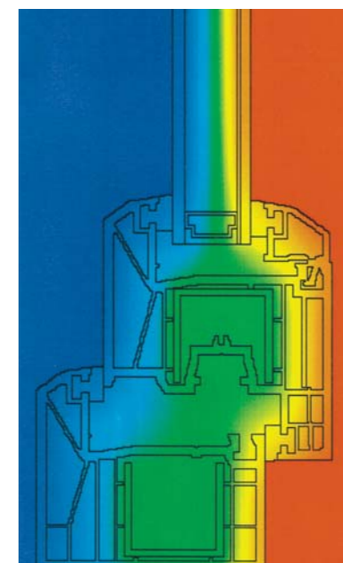
Toplotna izolacija: Temperaturna slika pokazuje optimalan tok izotermne krive.
